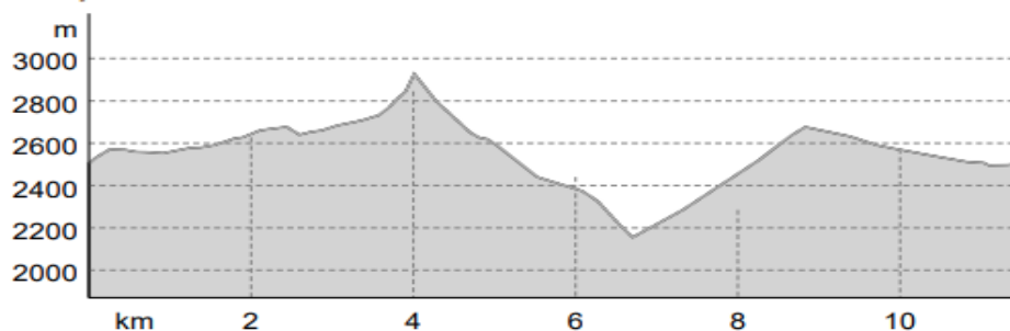
Höhenprofil
